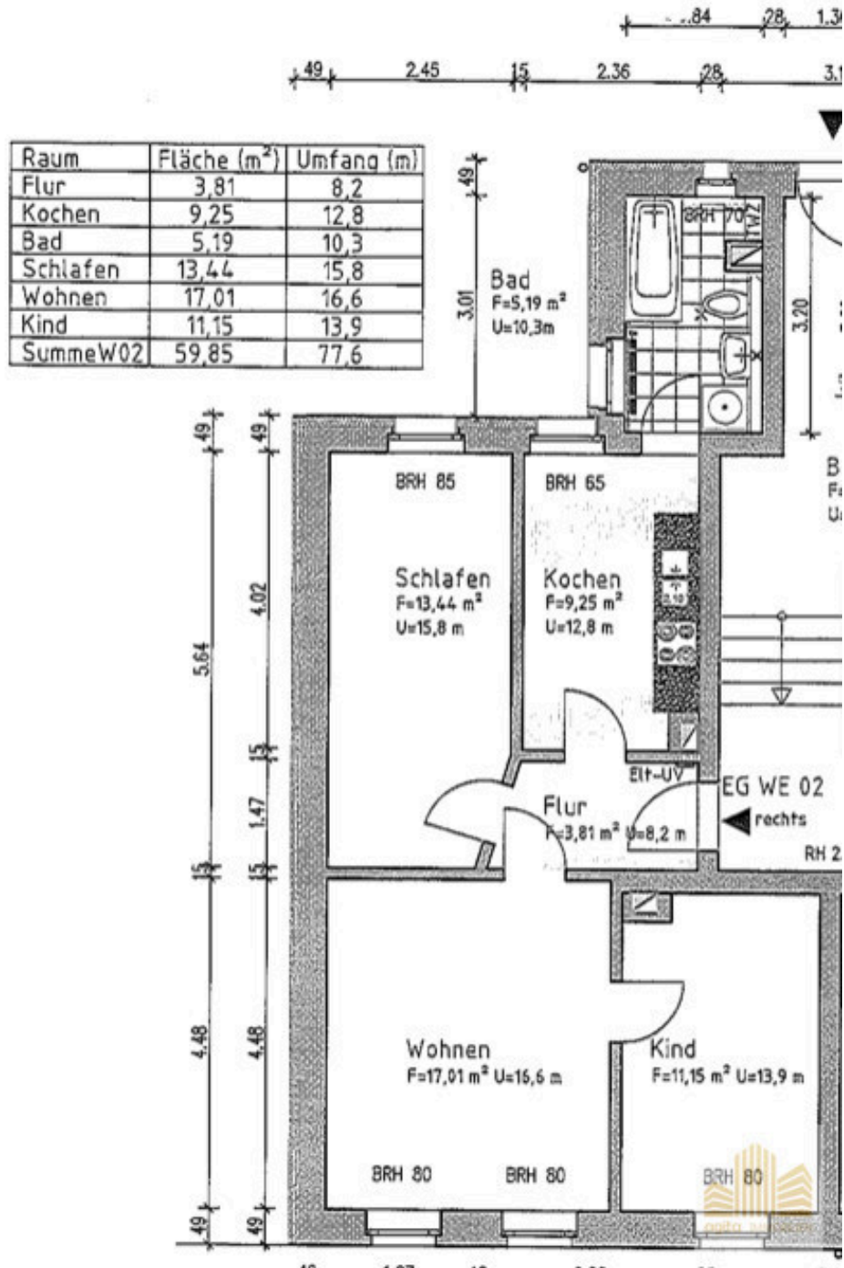
Grundriss
